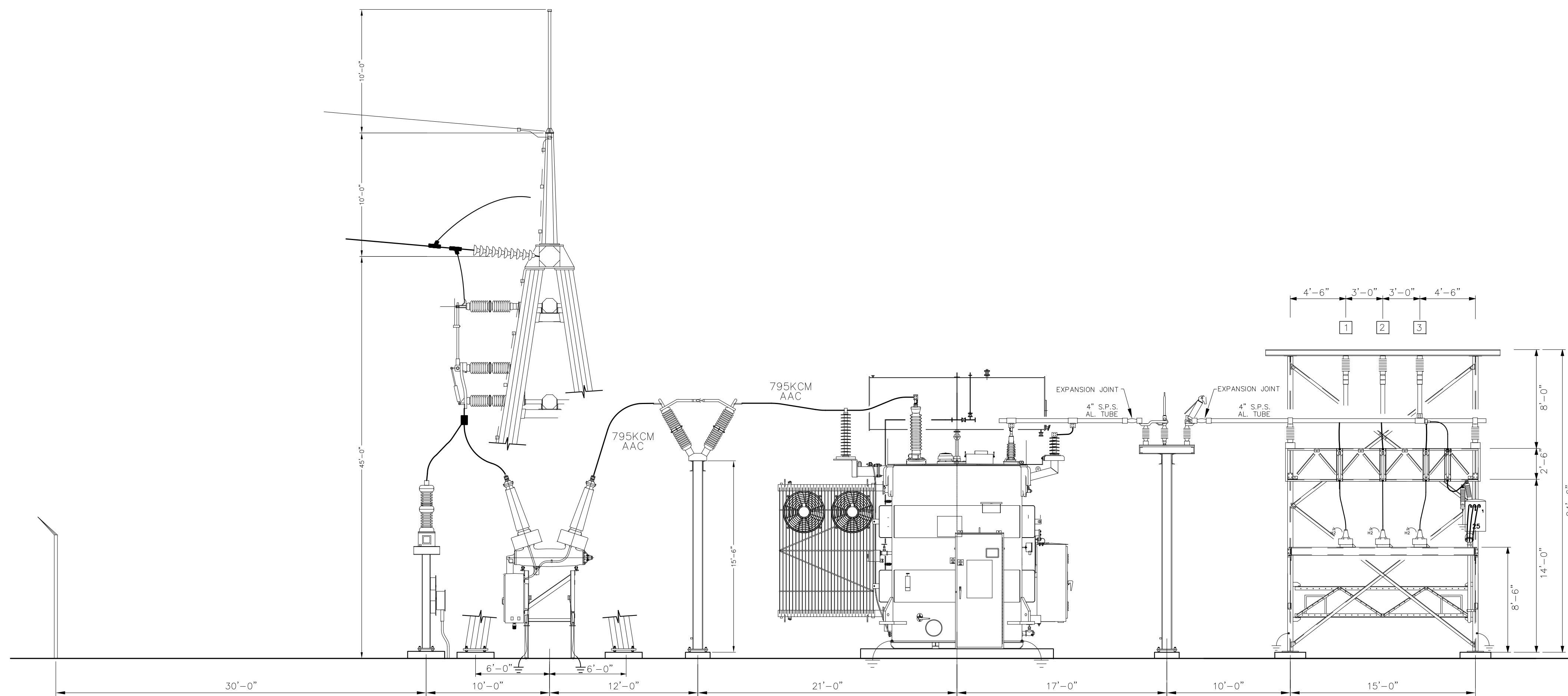
ELEVATION A-A
